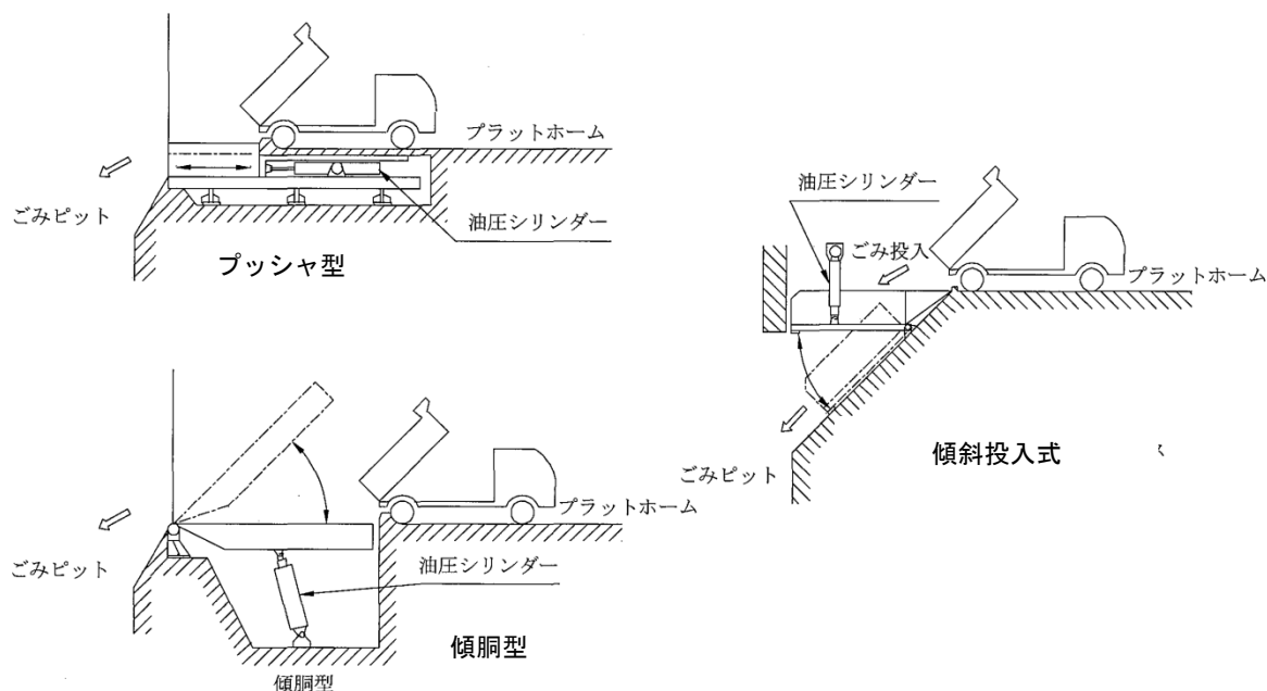
図 7-5 ダンピングボックスの投入方式例
