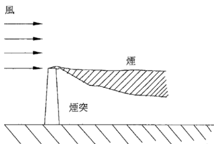
図 7-12 ダウンウォッシュ現象
