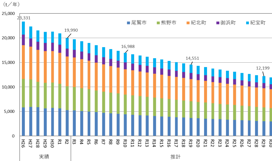
図 3-6 計画処理量の推移及び将来推計
