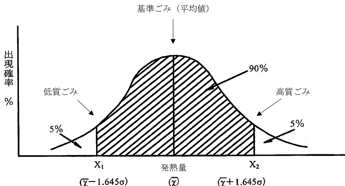
図 3-8 計画ごみ質設定における正規分布と 90%信頼区間
