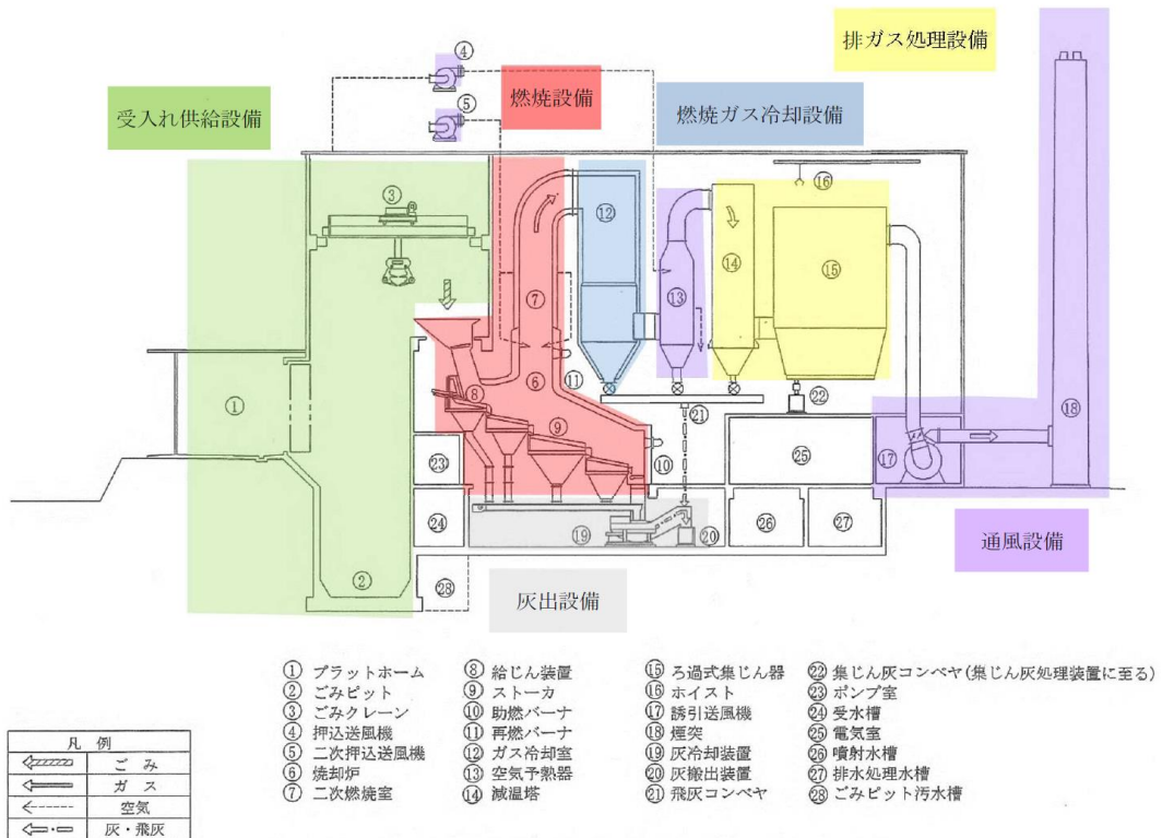
図 7-2 基本処理フロー（例）
