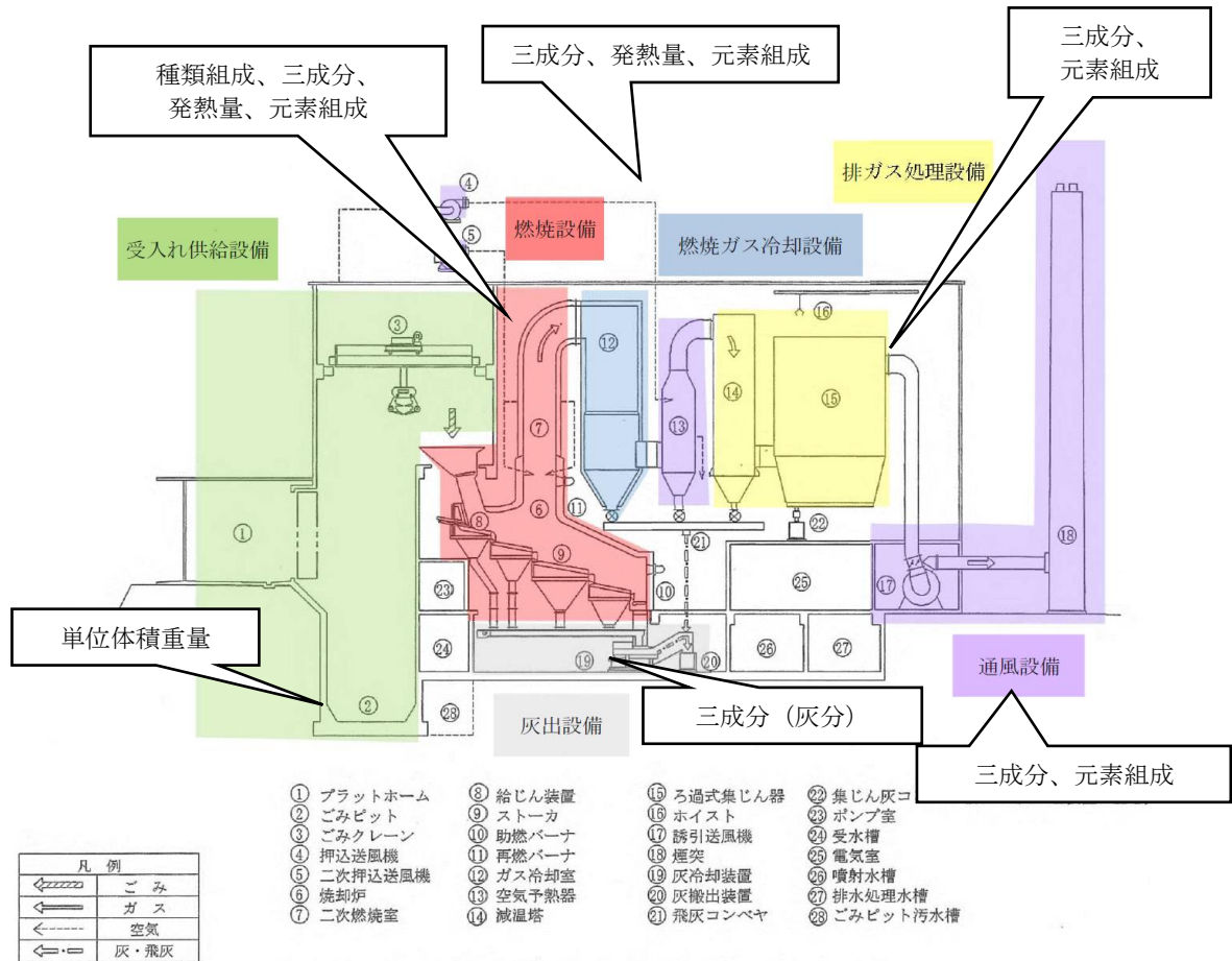
図 3-7 ごみ質と設備設計との関係性
