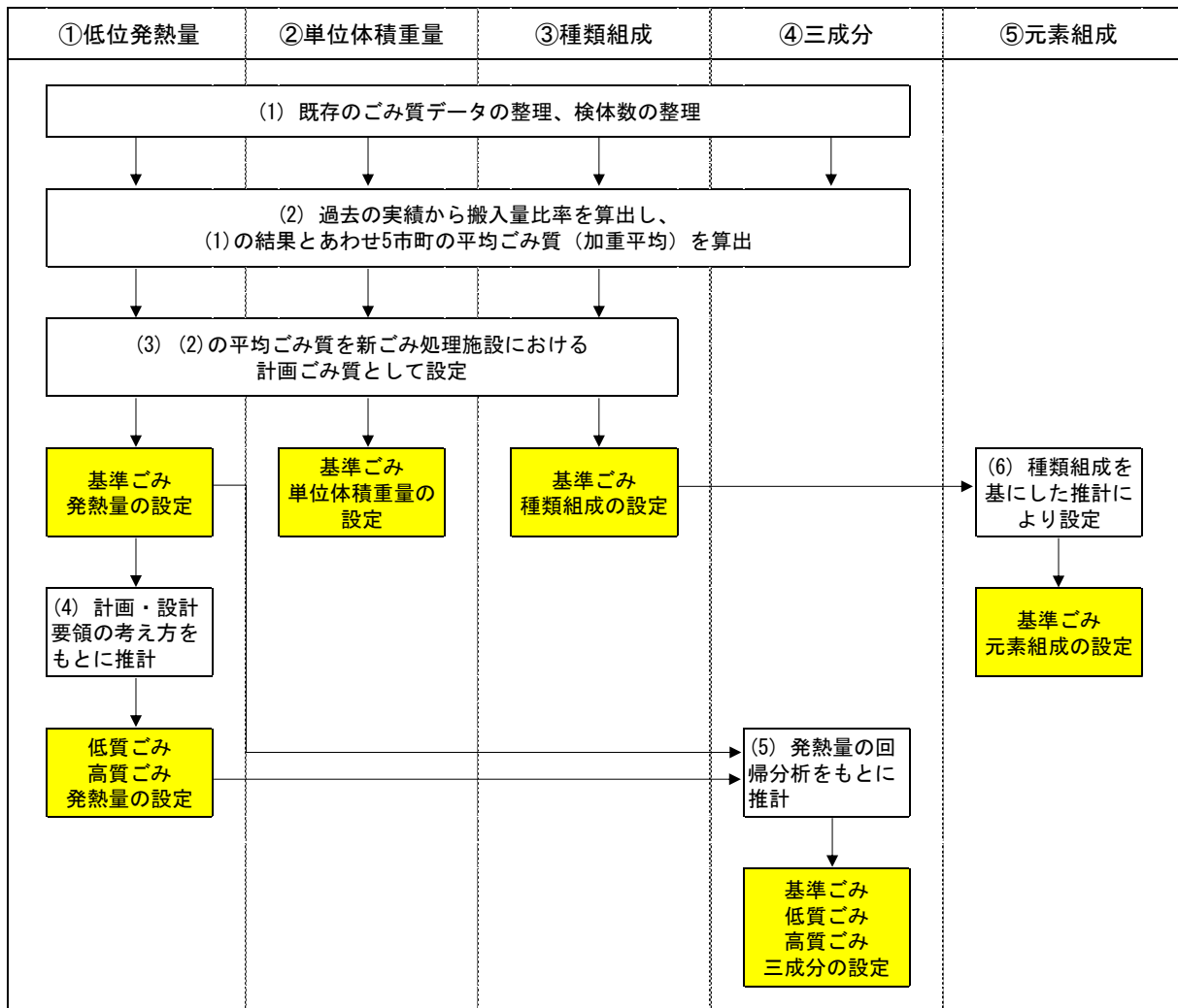
図 3-9 新ごみ処理施設における計画ごみ質の設定フロー
